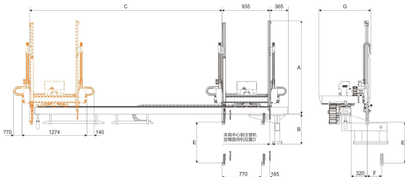
Outer Dimensions 尺寸图表
